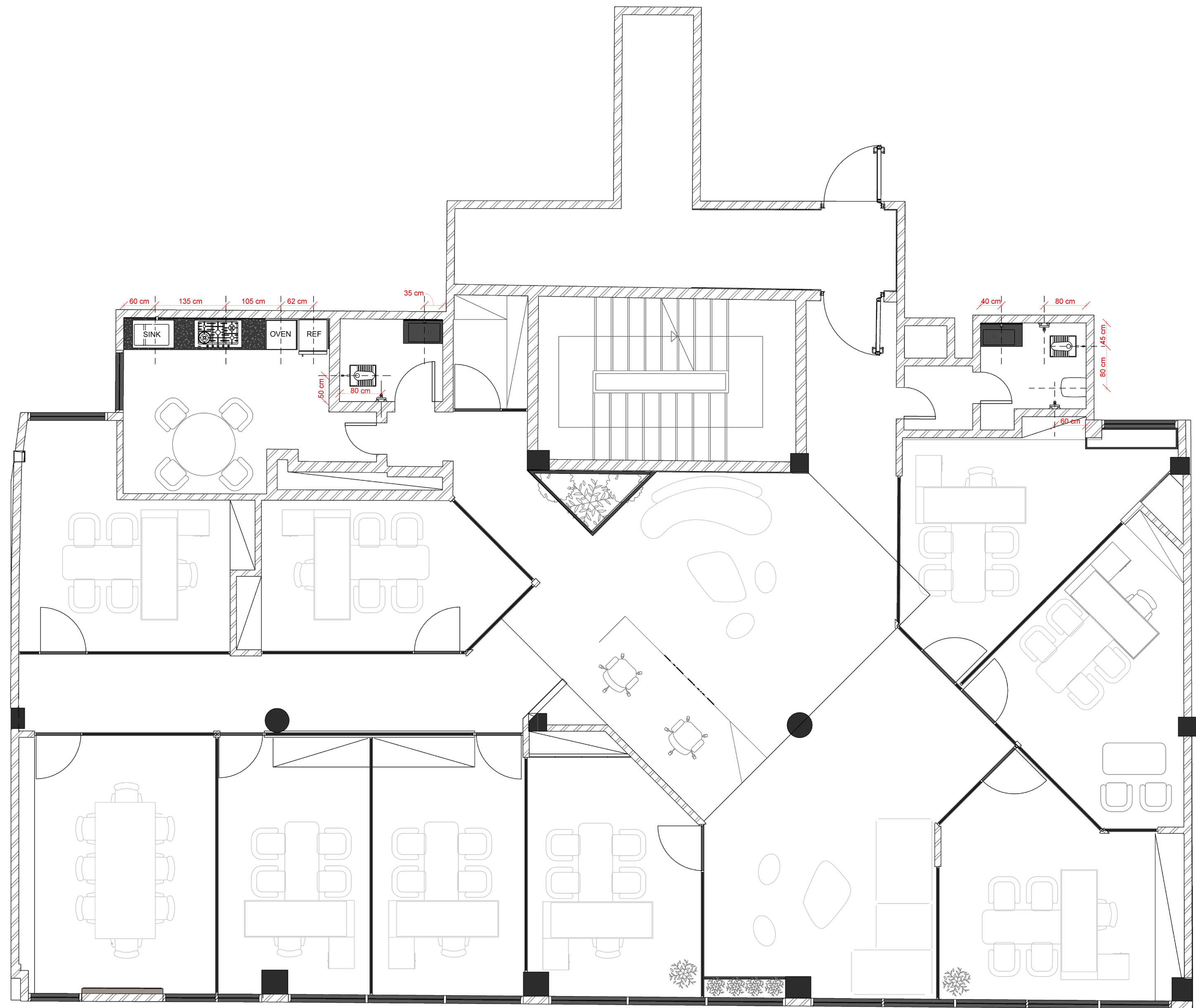
پلان جانمایی شیرآلات
