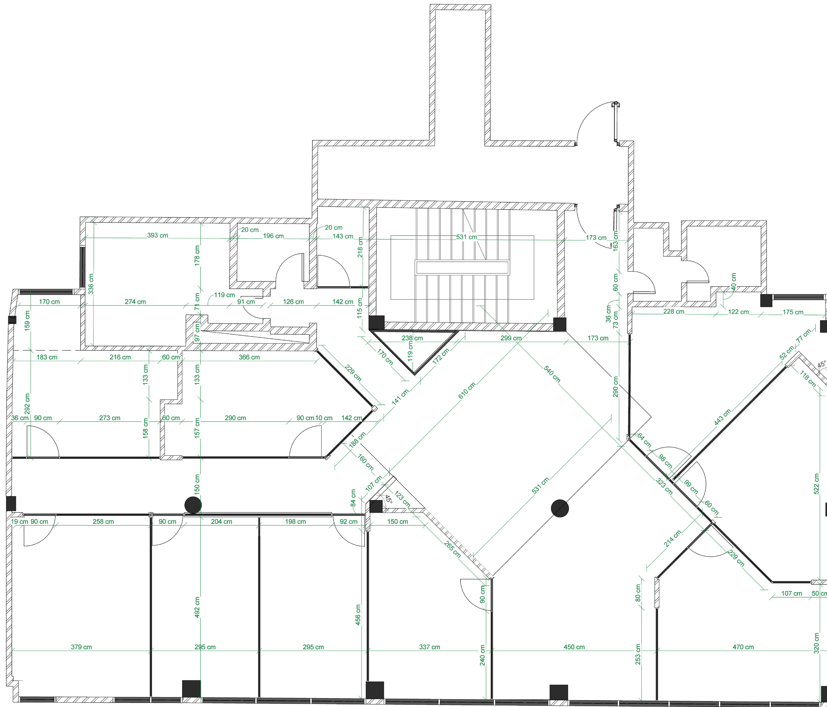
پلان اندازه گذاری - طبقه 04
