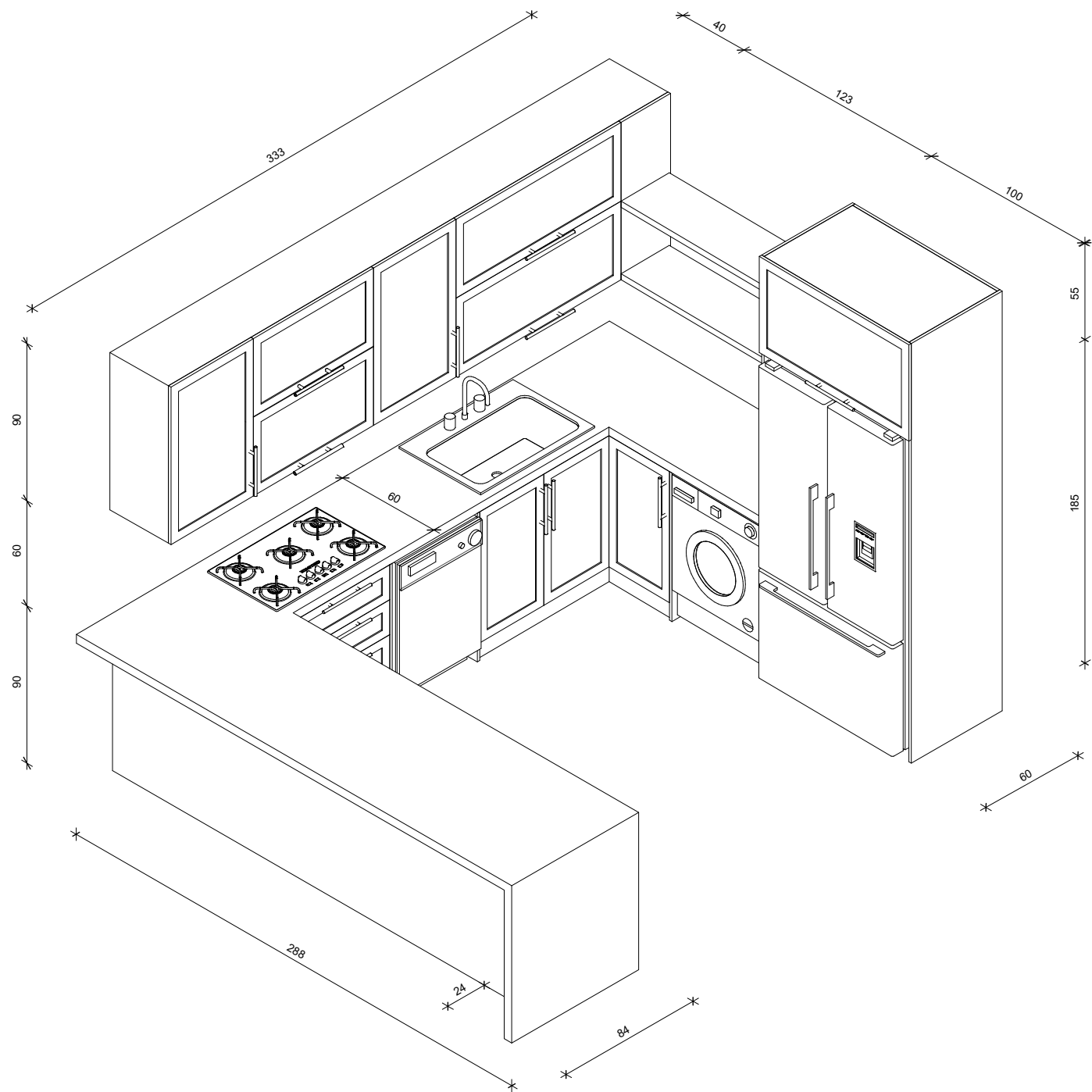
ایزومتریک آشپزخانه
