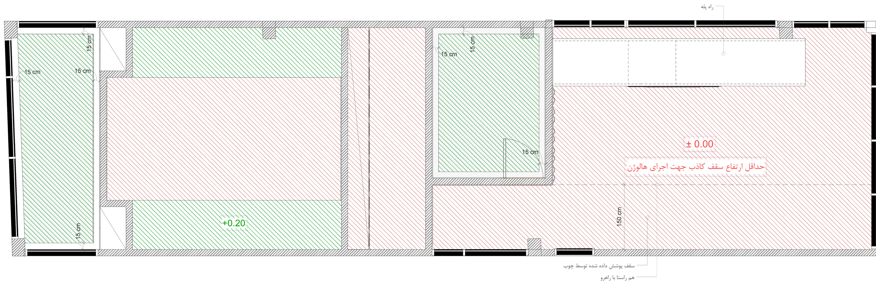
پلان سقف کاذب
