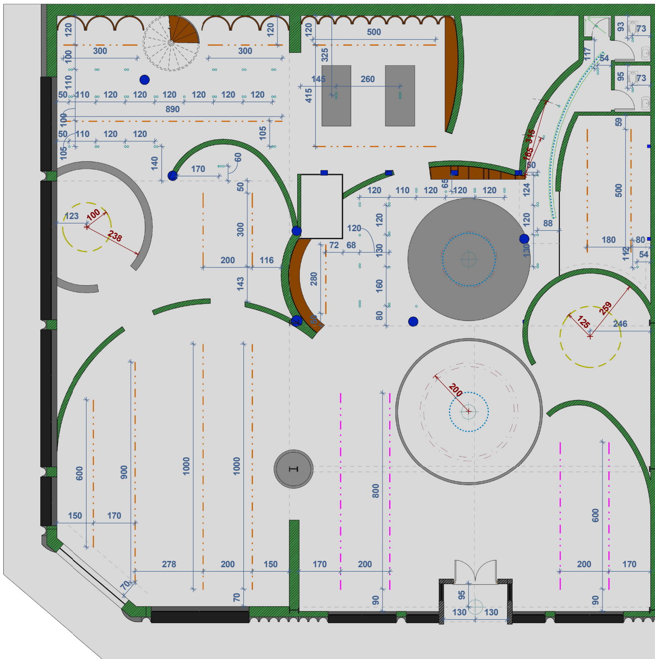
پلان نور پرودازی سقف
