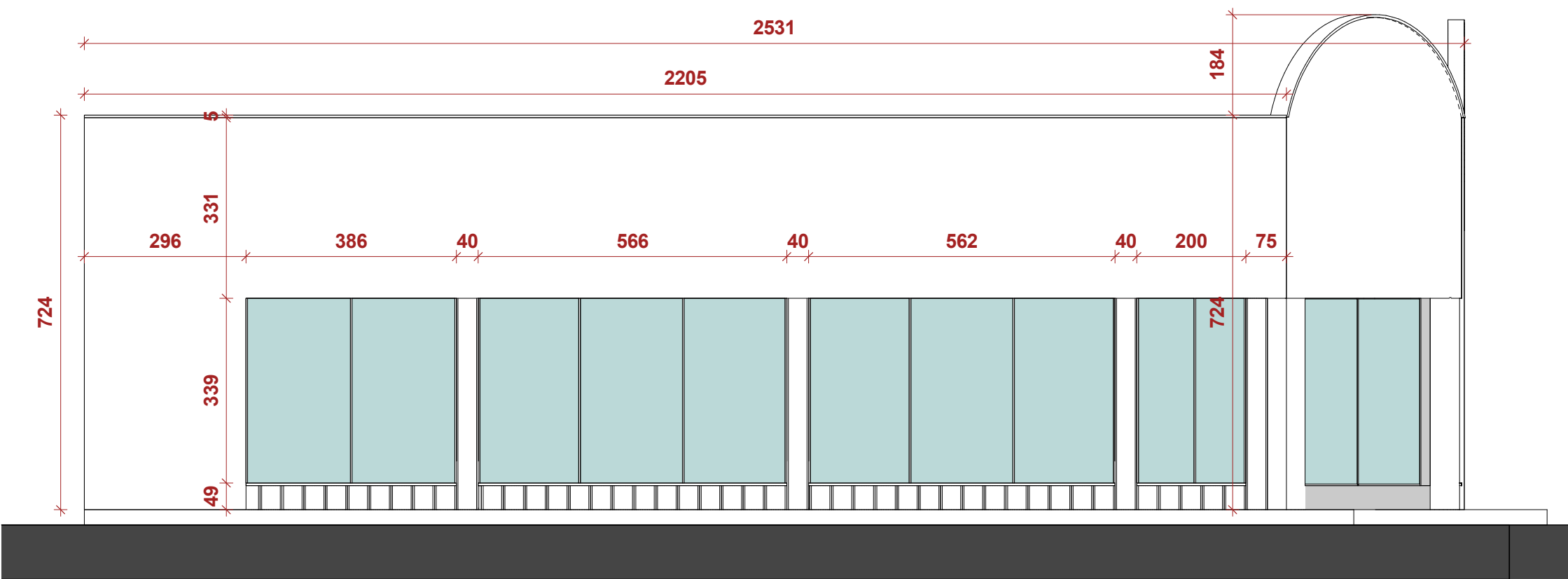
نمای جانبی
