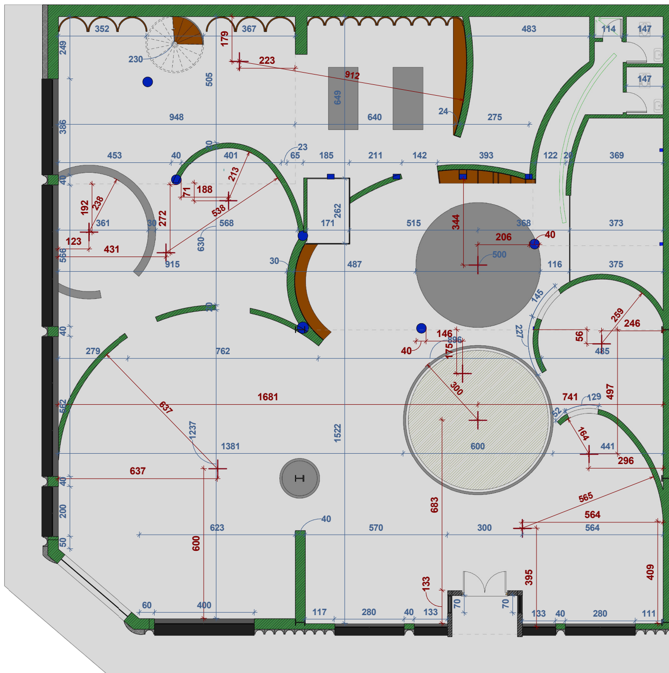
پلان تیغه چینی
