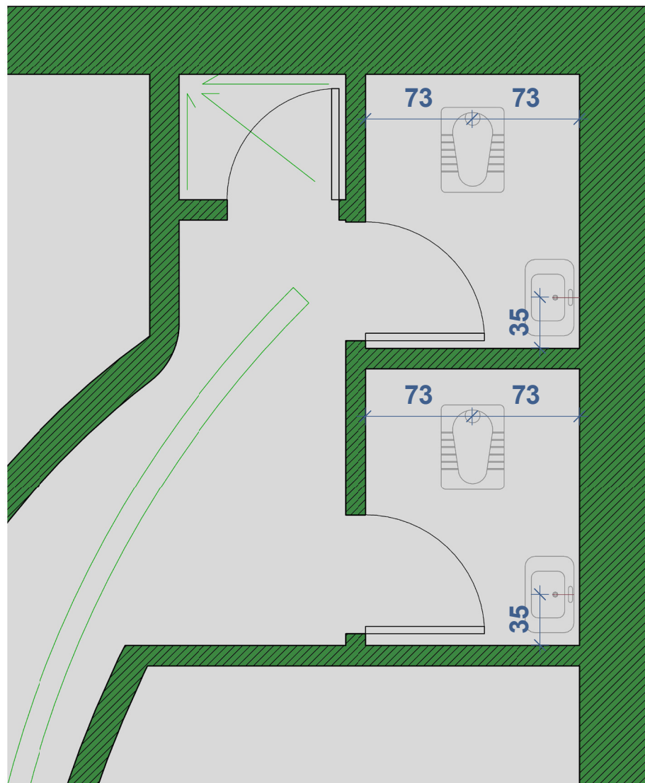
جانمایی شیرآلات
