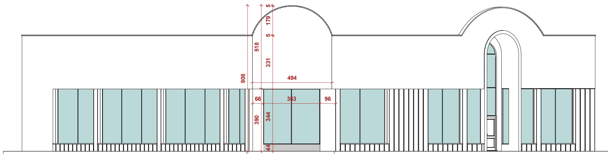
نمای مورب
