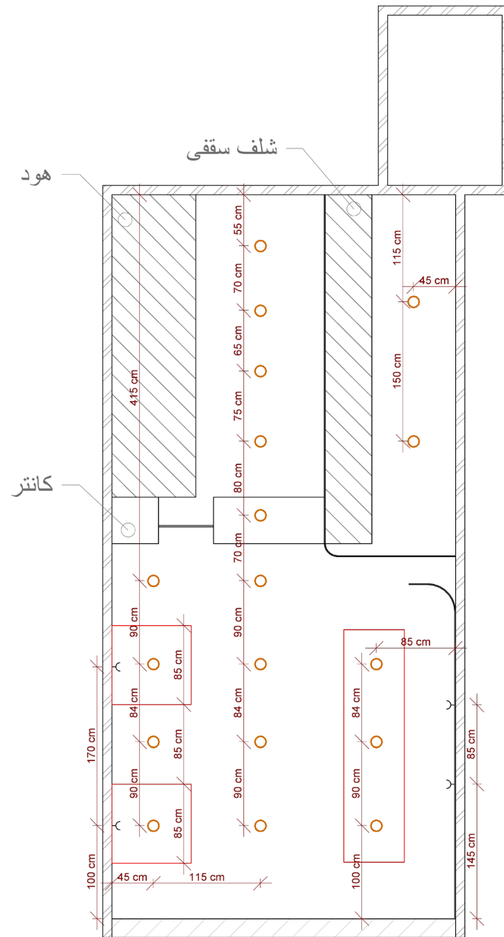
پلان نورپردازی و پریرها
