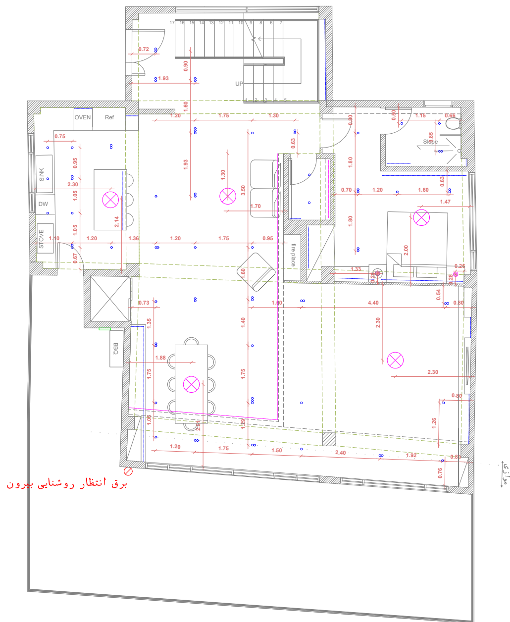
پلان همکف - اندازه گذاری روشنایی
