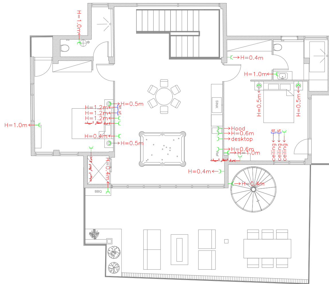
پلان پیریزهای اول
