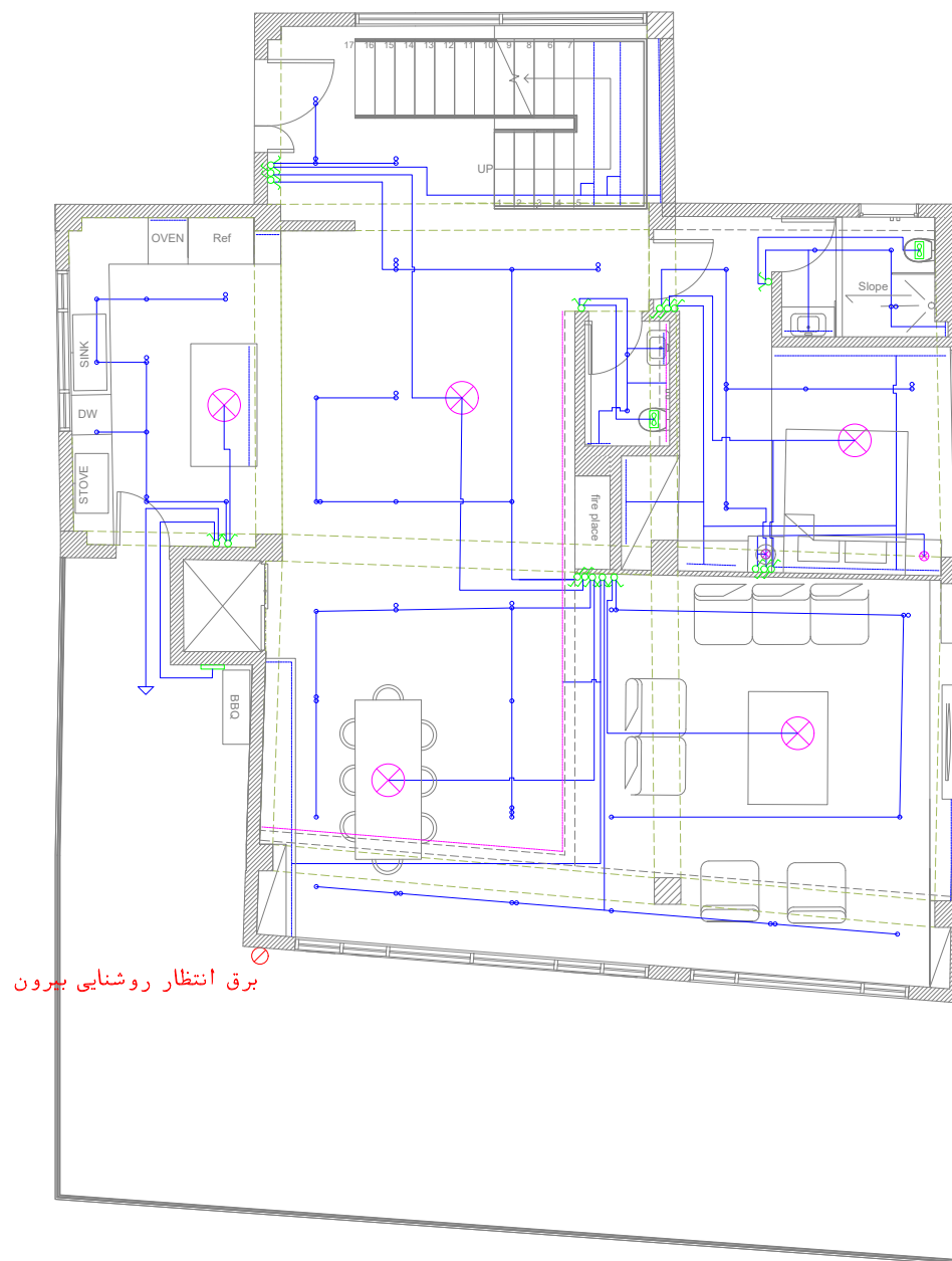
پلان کلیدهای همکف
