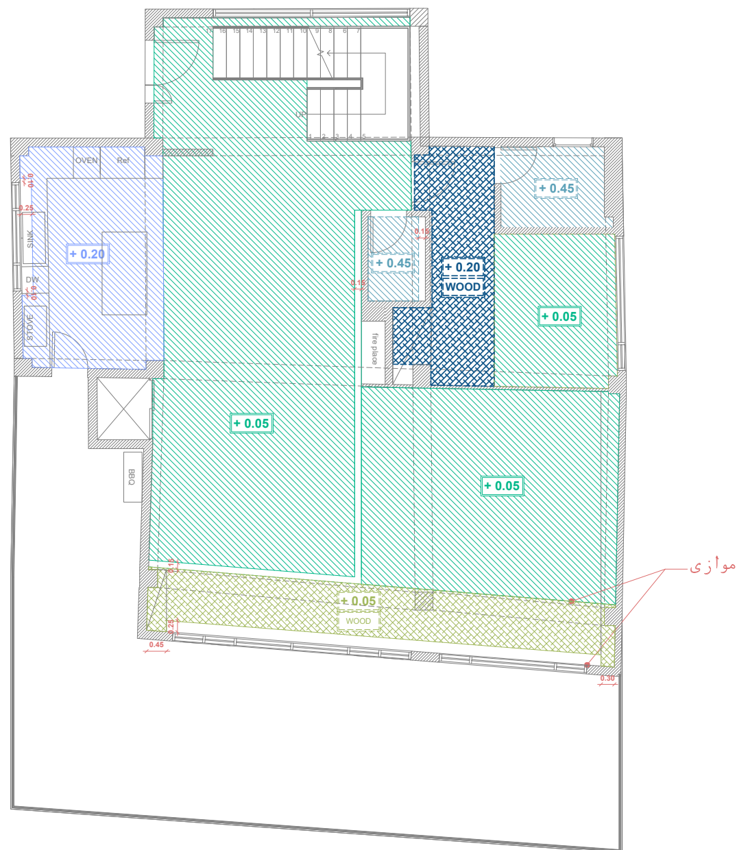
پلان همکف-سقف کاذب
