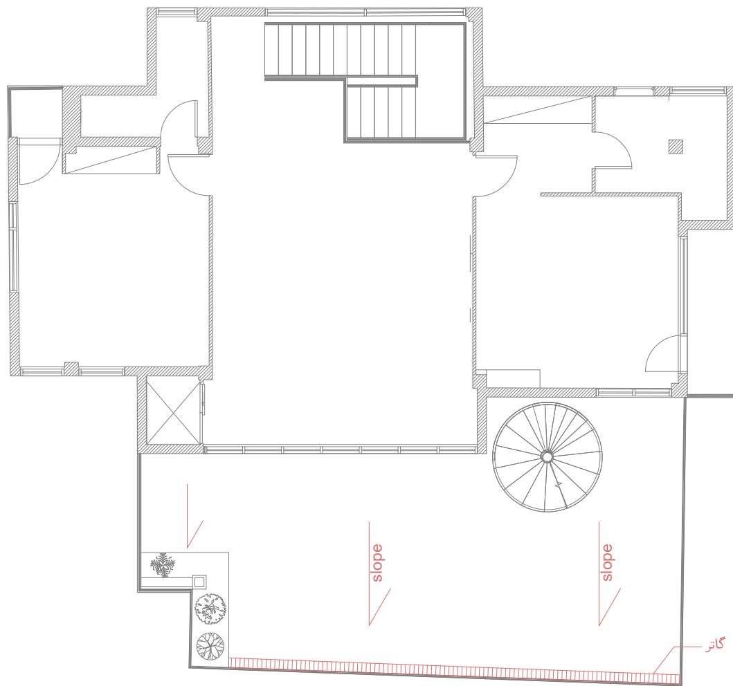
پلان شیب بندی تراس
