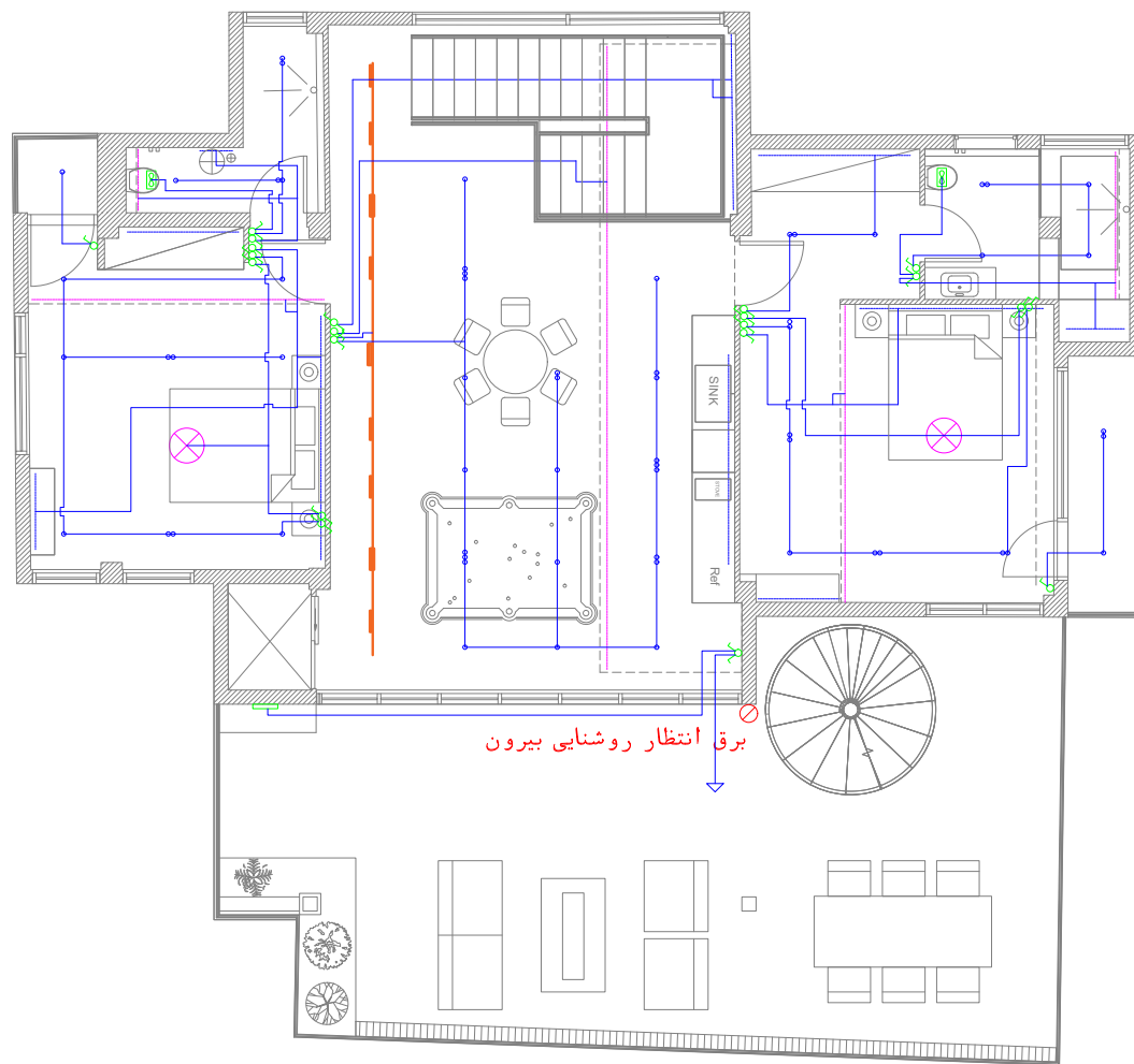
پلان کلیدهای اول
