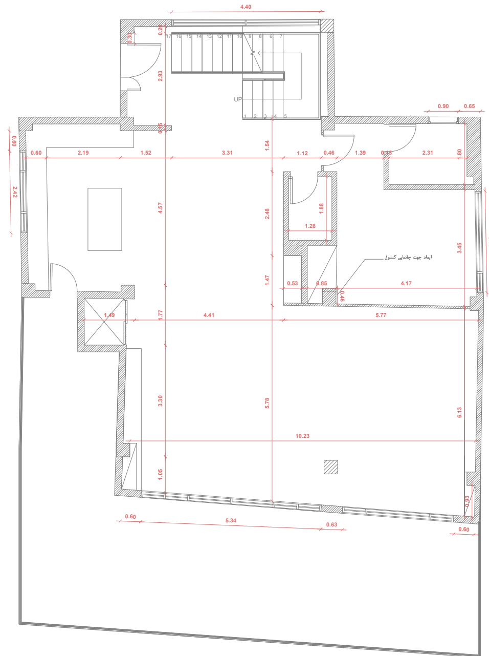
پلان اندازه گذاری همکف
