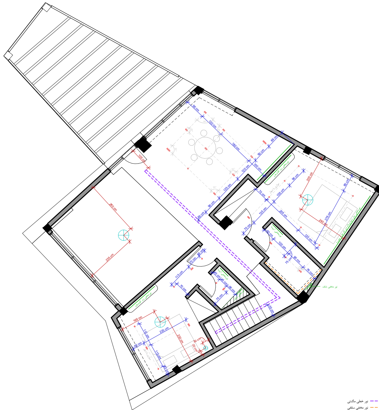
پلان نورپردازی - طبقه اول
