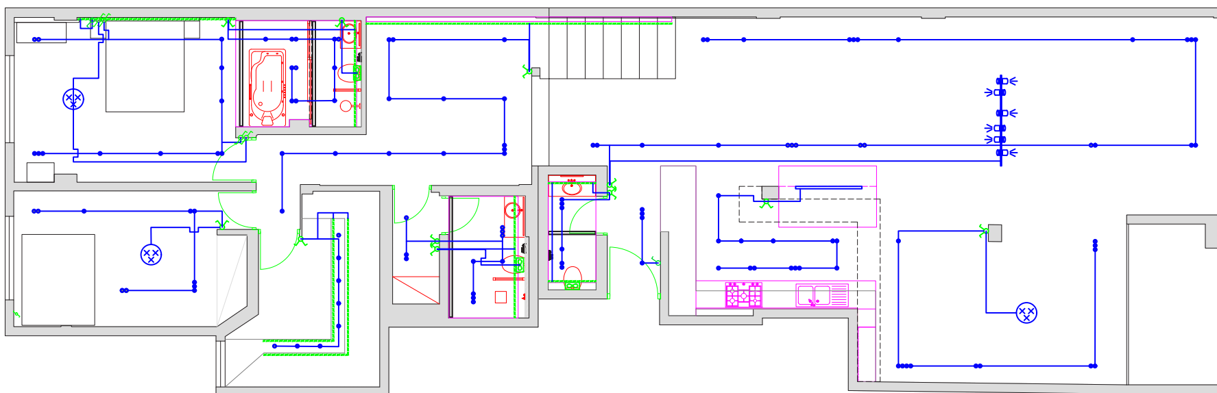
جانمایی کلید بوکان
