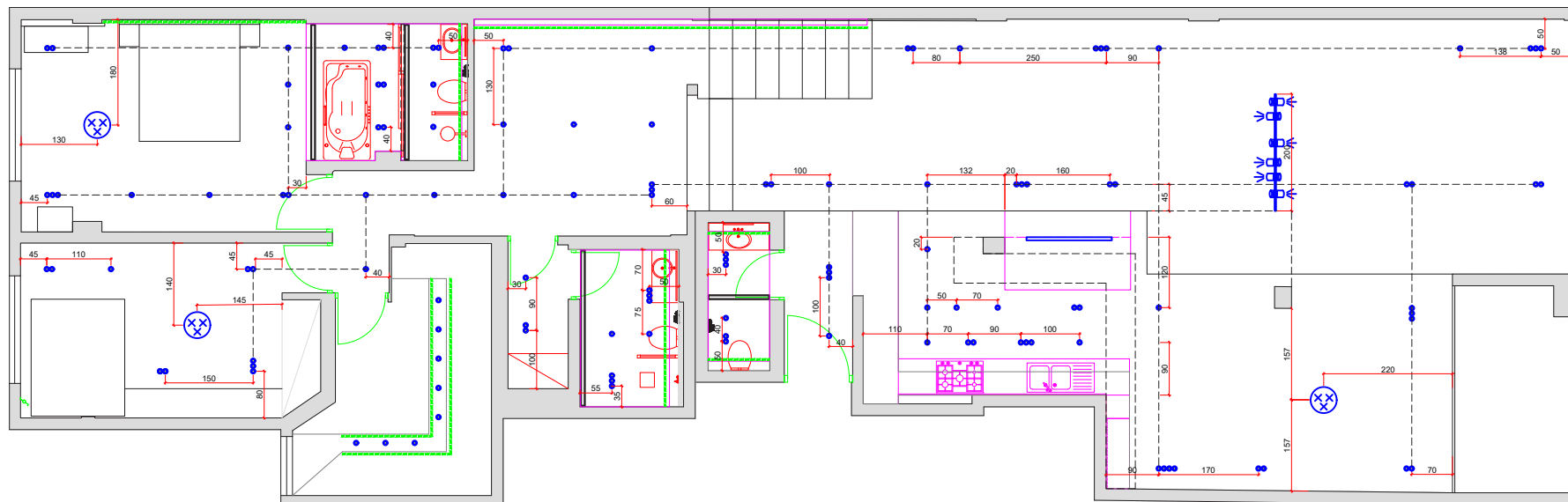
جانمایی روشنایی بوکان
