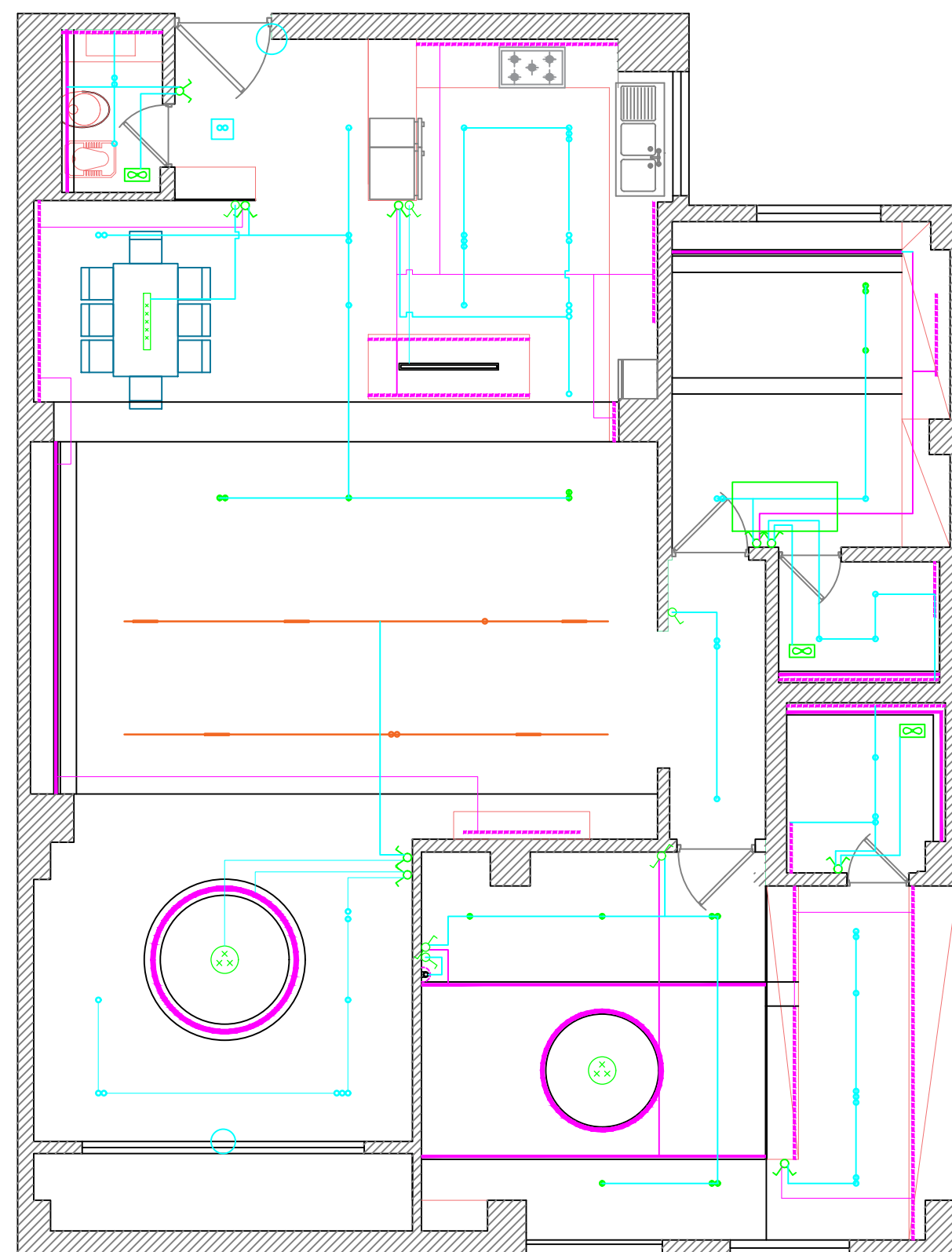
پلان کلید و سیم کشی
