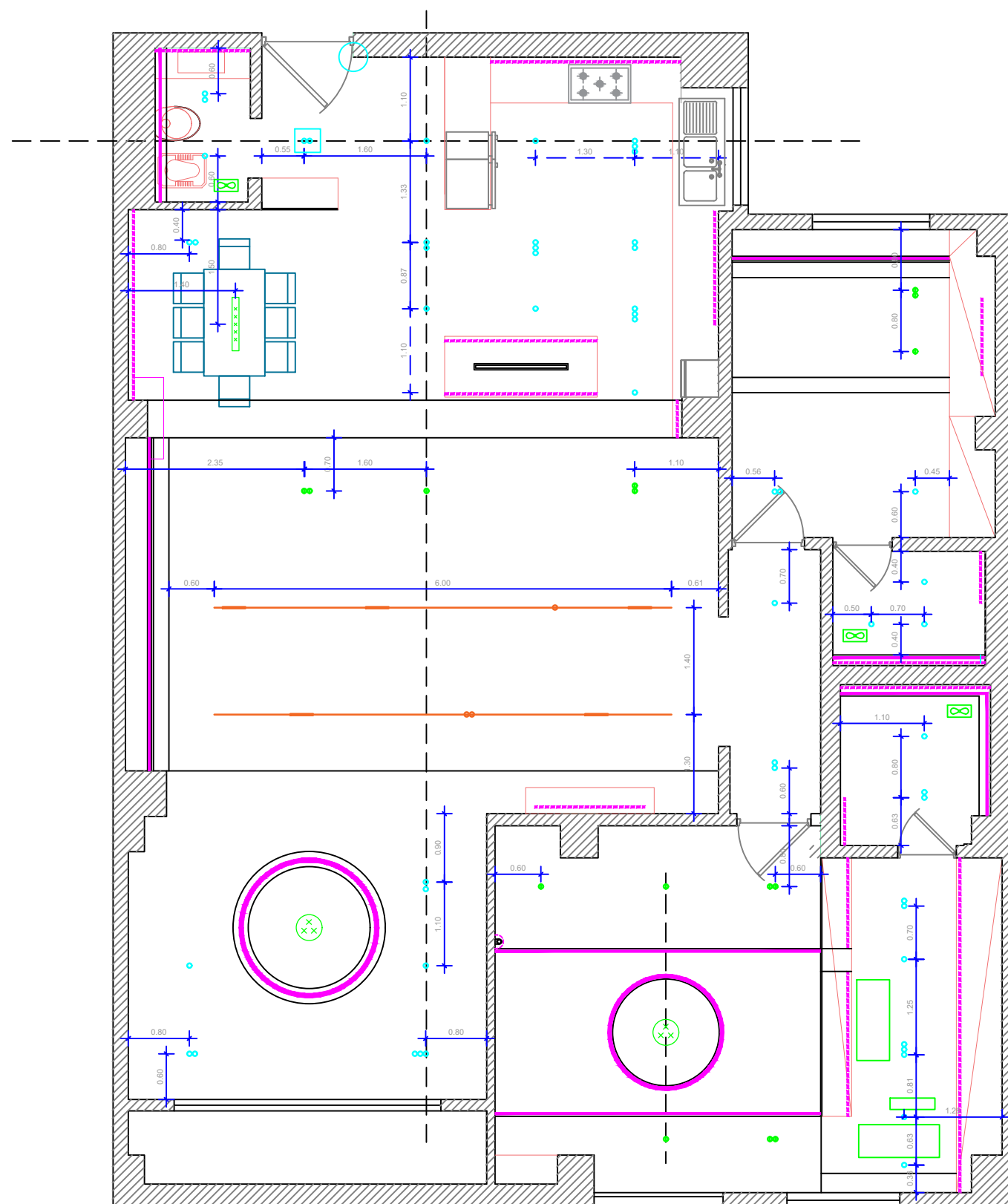
پلان اندازه گذاری روشنایی
