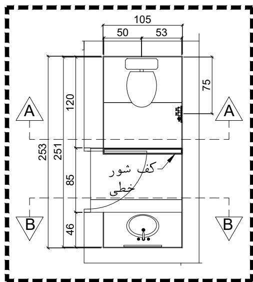
پلان سرویس بهداشتی
