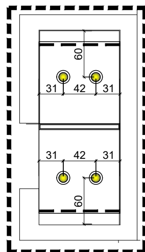
پلان منعکس سقف
