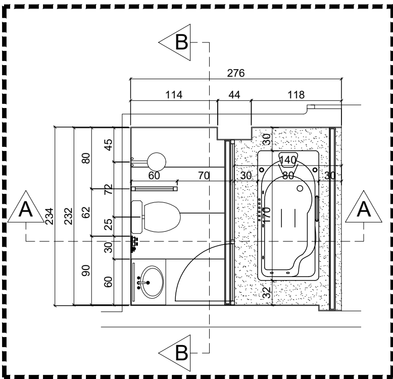
پلان سرویس مستر
