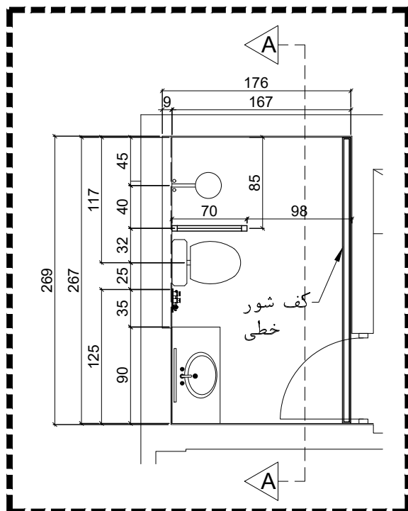
پلان سرویس بهداشتی
