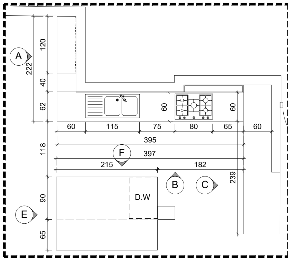
پلان کف آشپزخانه
