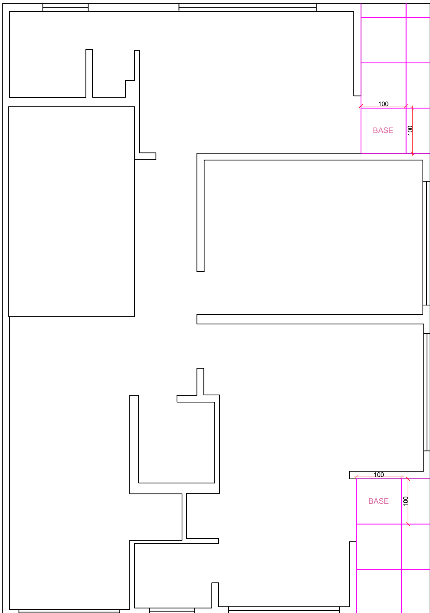
پلان سرامیک بالکن
