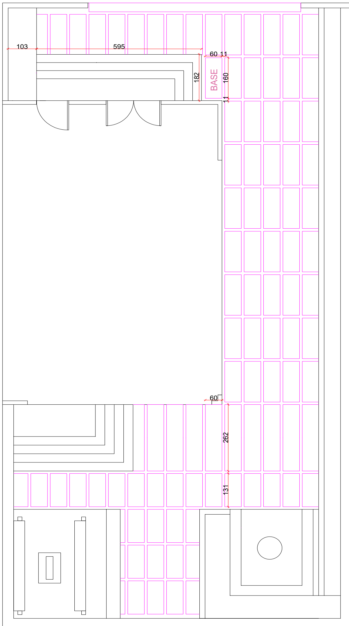
پلان کف سازی محوطه
