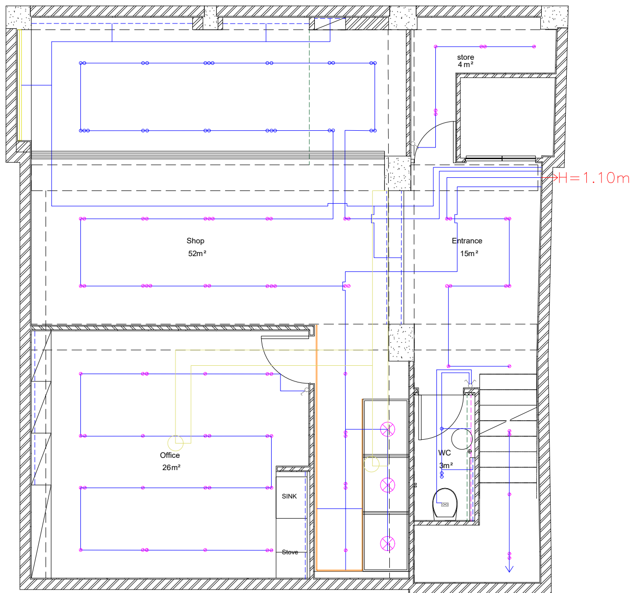
طبقه ۱ - پلان کلید های روشنایی
