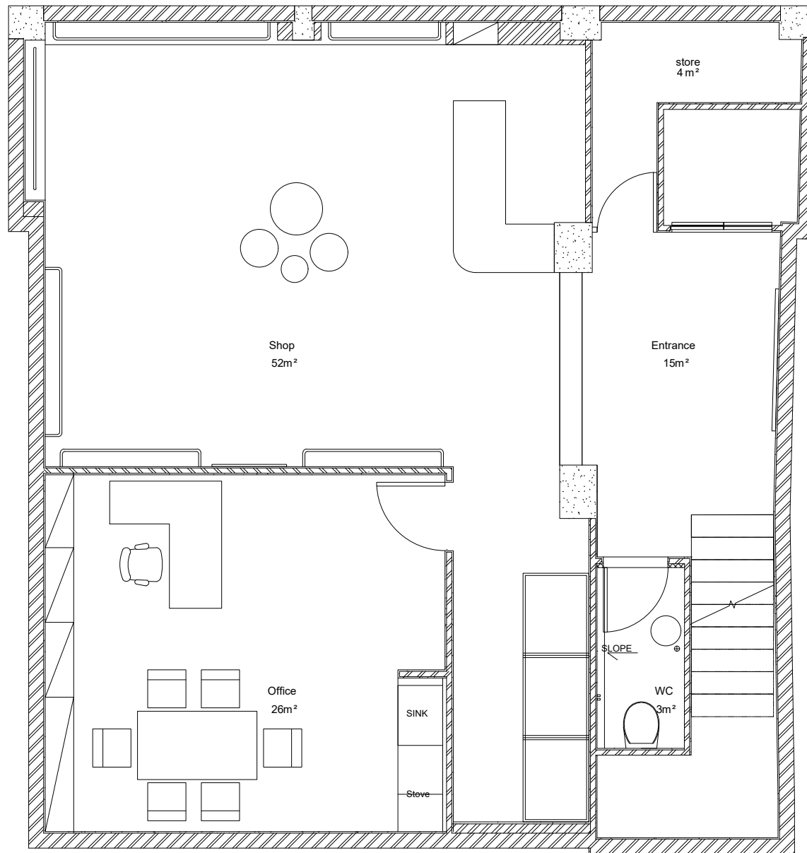
طبقه ۱ - پلان مبلمان
