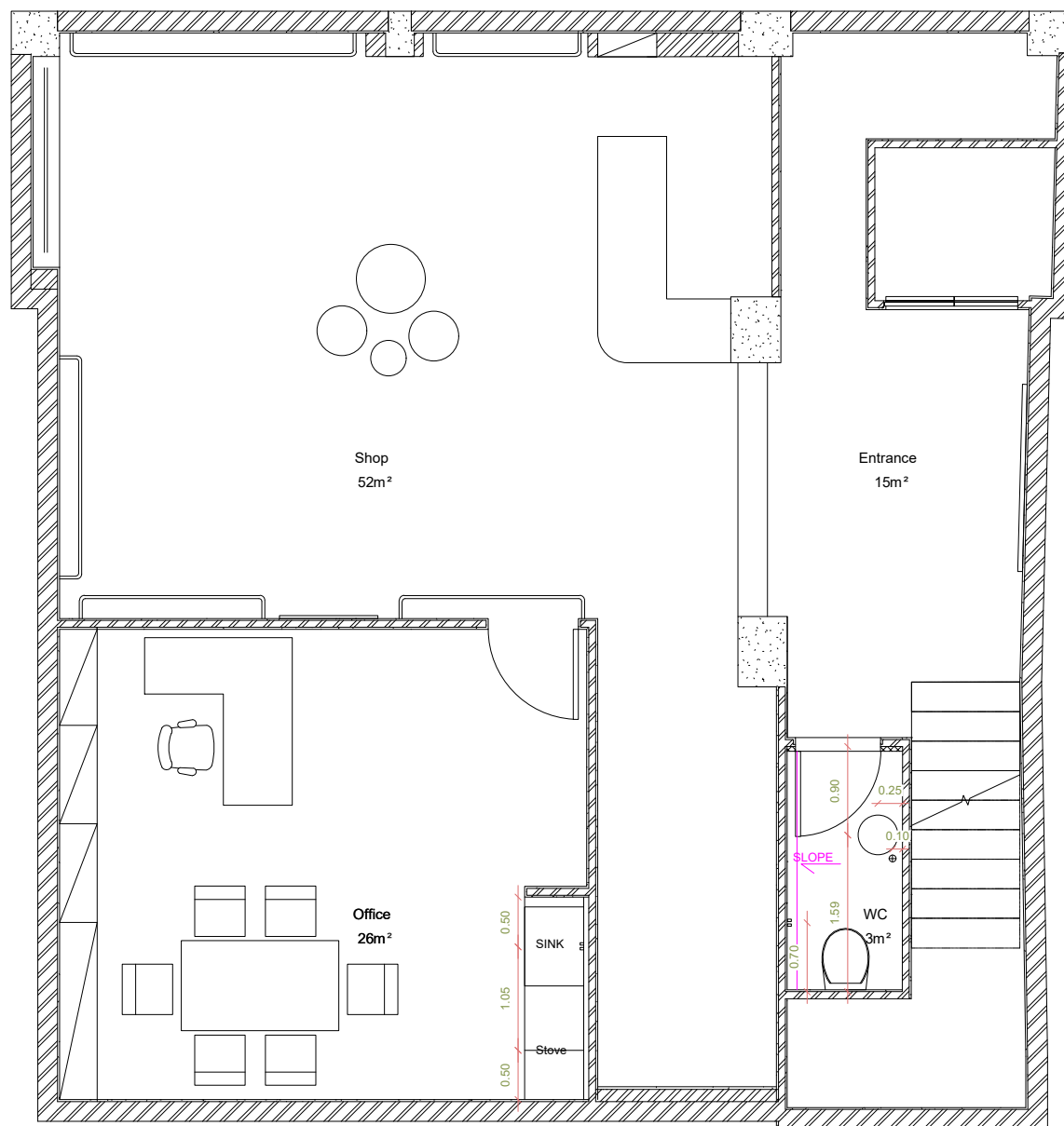
طبقه ۱ - پلان جانمایی شیر آلات
