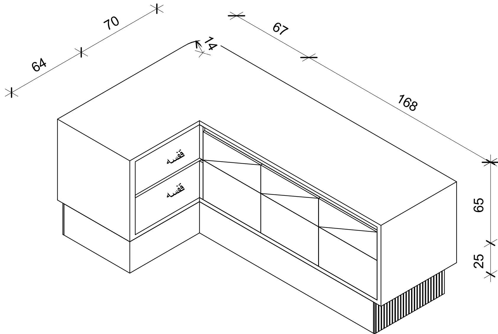
ایزومتريک صندوق
