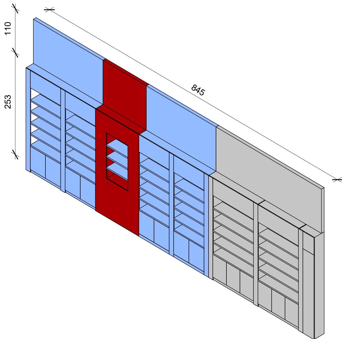
ایزومتريک قفسه شمالي فروشگاه
