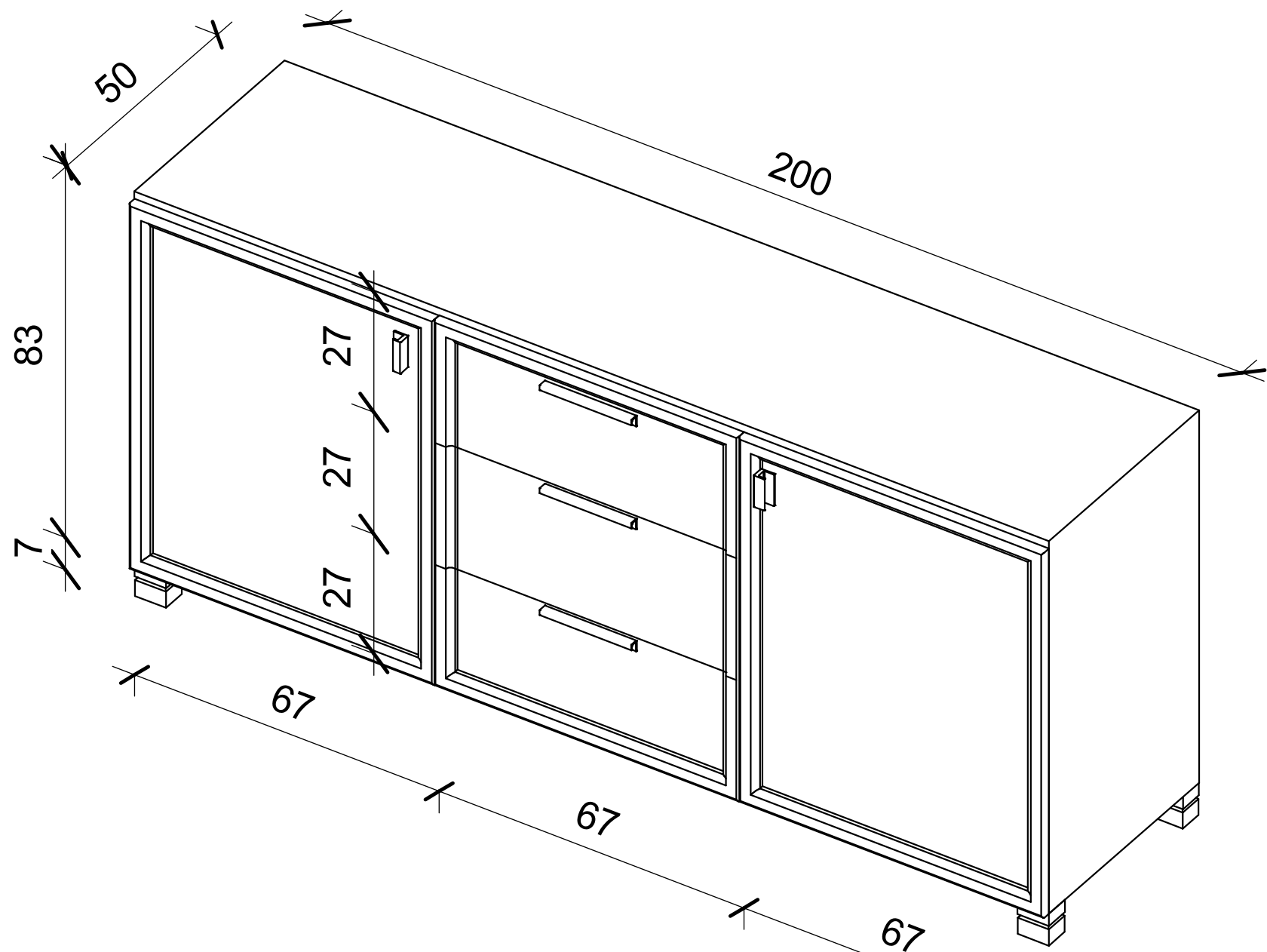
ایزومتریك كنسول سالن
