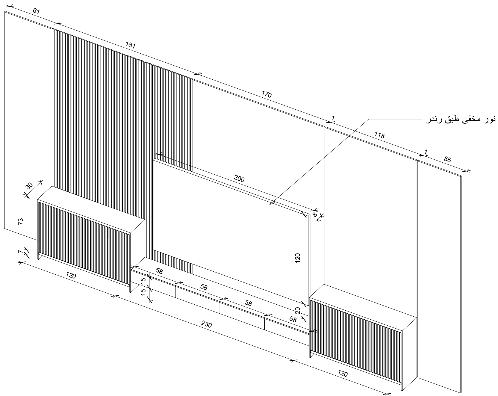
ایزومتریک تی وی وال
