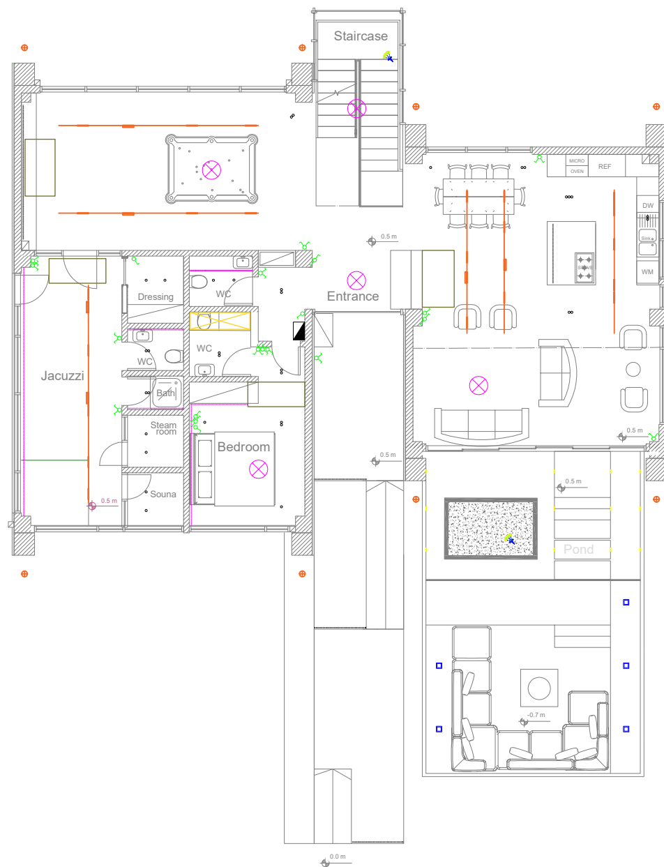
پلان جانمایی کلید های روشنایی همکف
