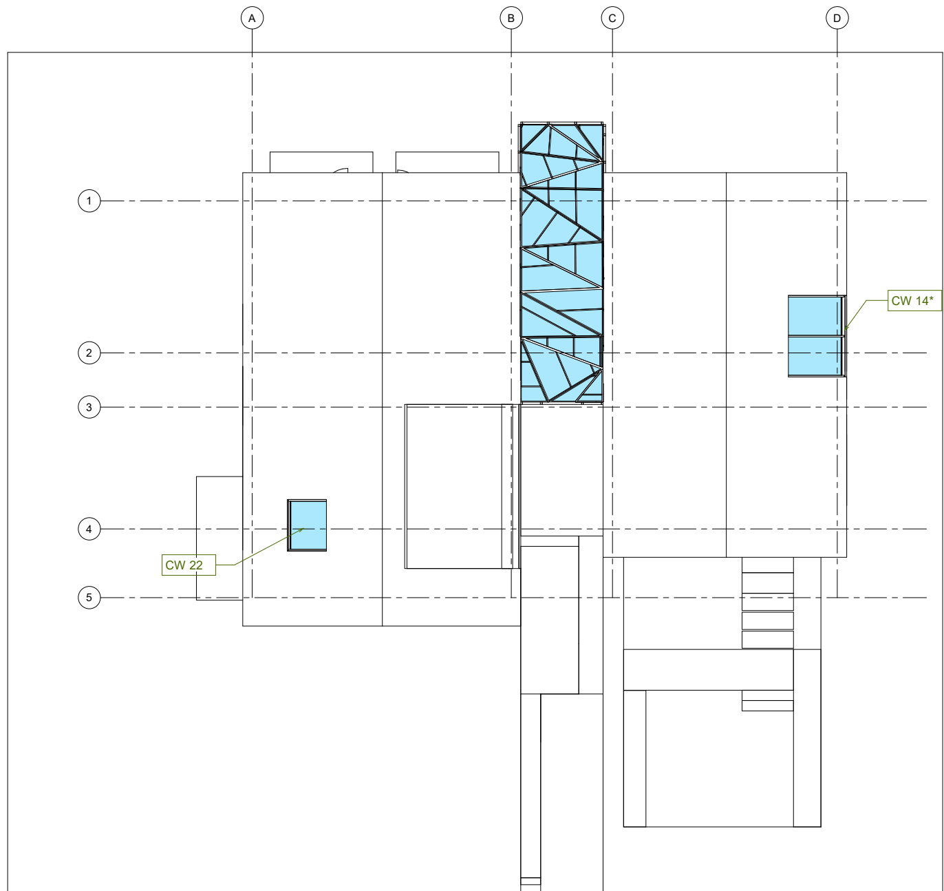
پلان نام گذاری کرتین وال - بام
