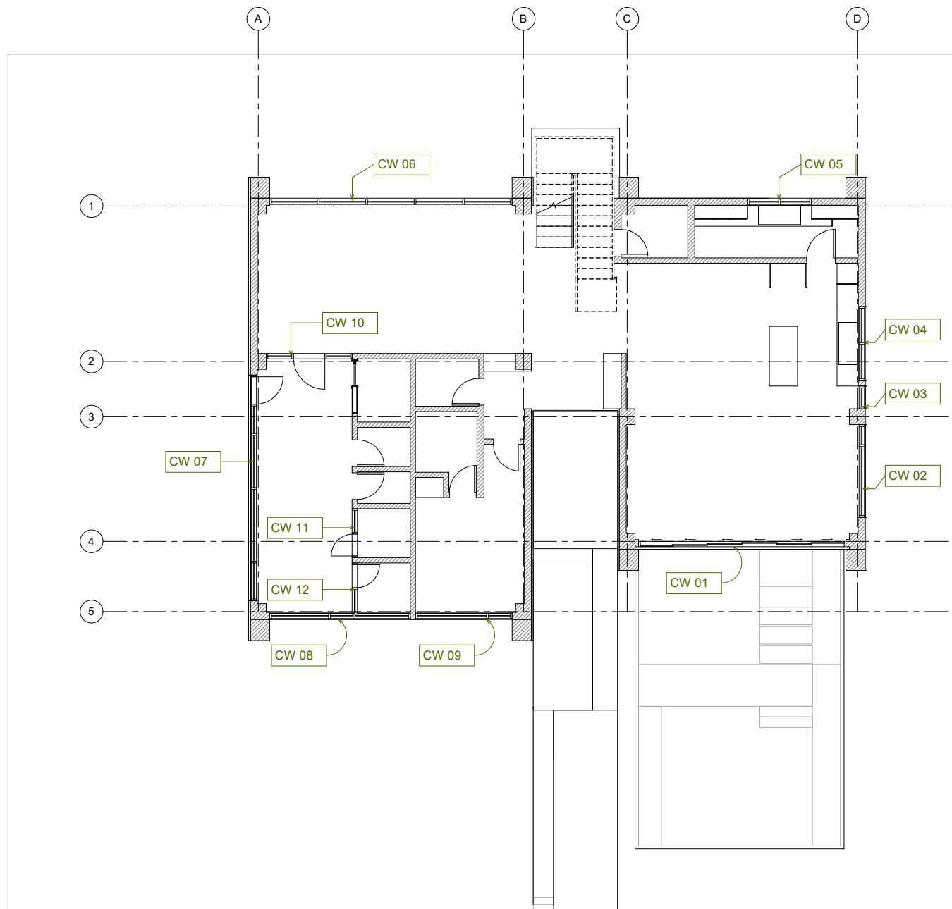
پلان نام گذاری کترین وال - همکف
