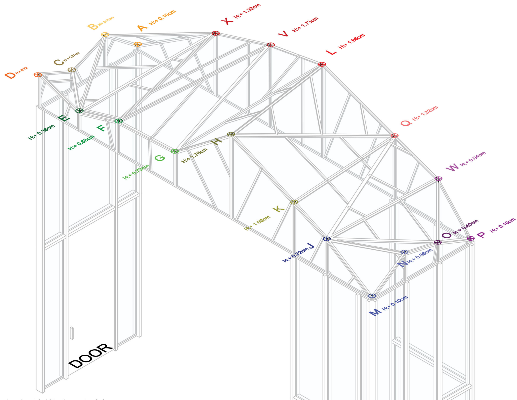
جانمایی ایزومتریک نقاط پارامتریک سازه شیشه ای راه پله
