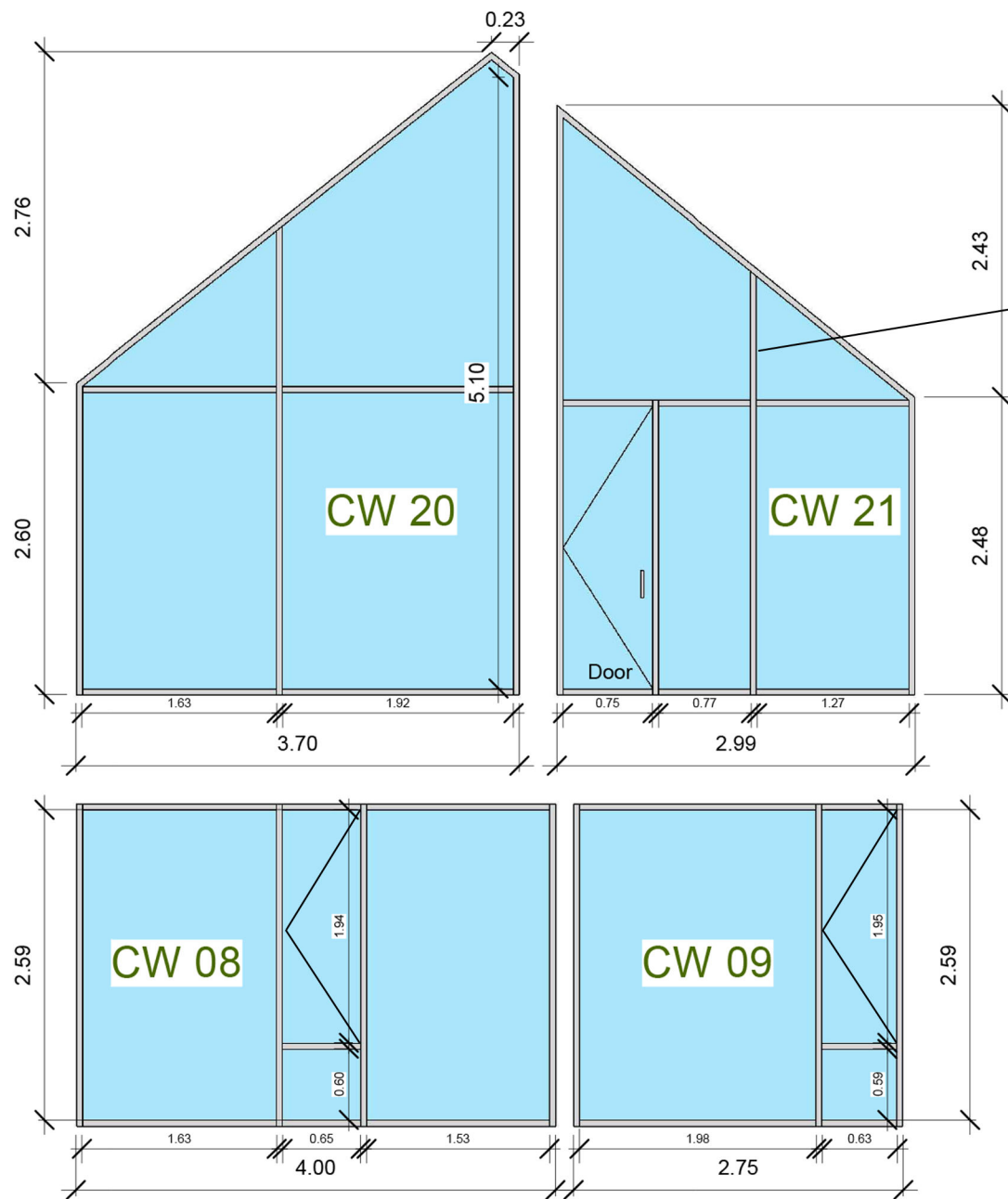
نمای جنوب شرقی
