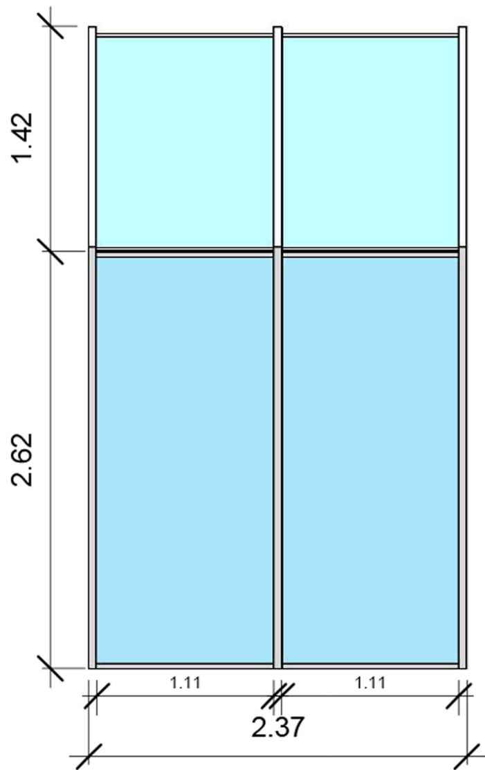
نمای شمال شرقی
