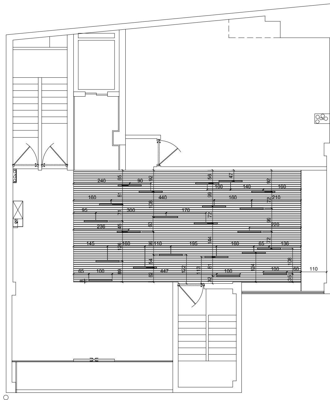
پلان جانمایی لامپ های خطی (روکار)
