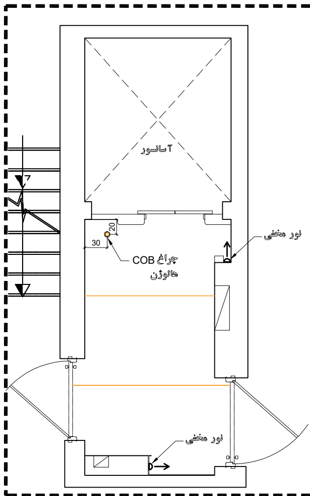
پلان جانمایی منابع نور
