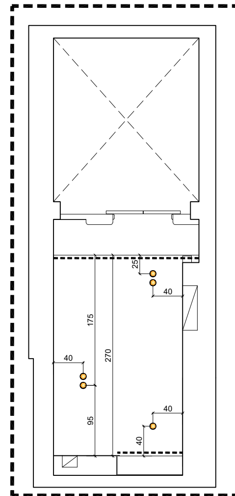
پلان منعکسی شده سقف
