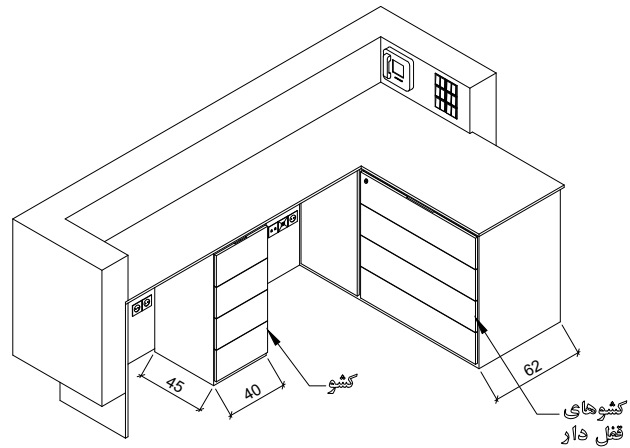
نمای ایزومتریک
