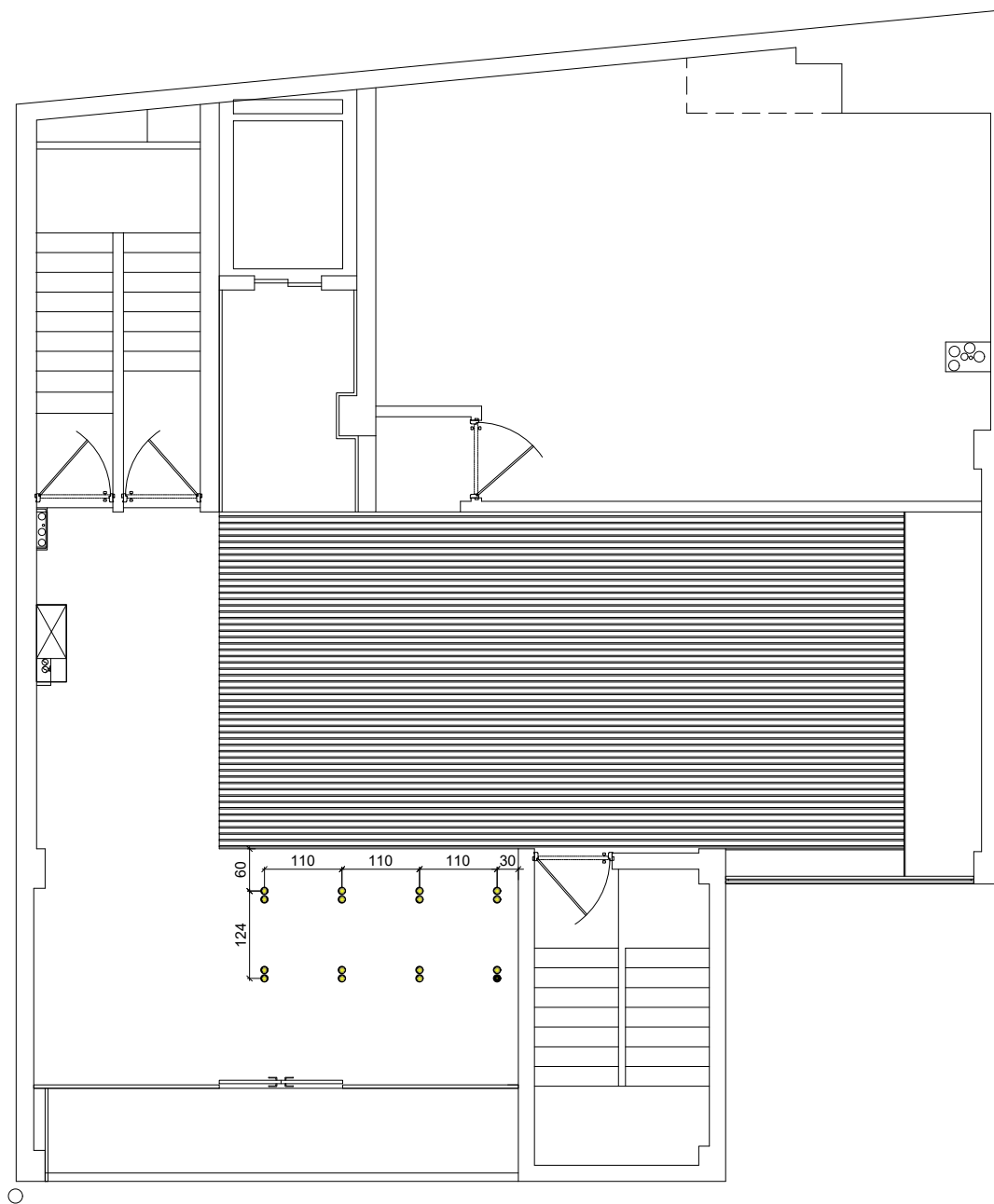
پلان جانمایی لامپ های سقفی تو کار (هالوژن)
