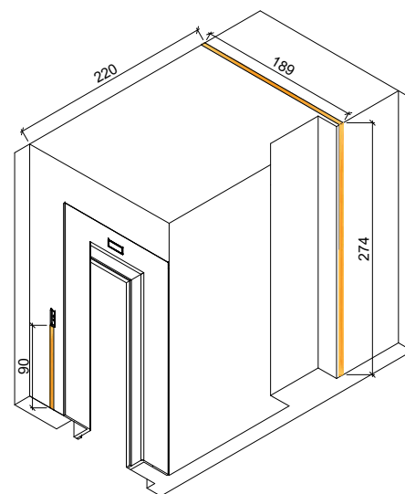
ورودی آسانسور
