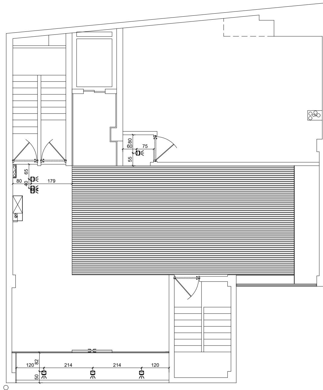
پلان جانمایی لایپ های سقفی تو کار (هالوژن)
